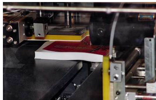
Der pneumatische Aufbau des FKS/Challenge-Dreiseitenschneiders sorgt für präzise Buchergebnisse.
